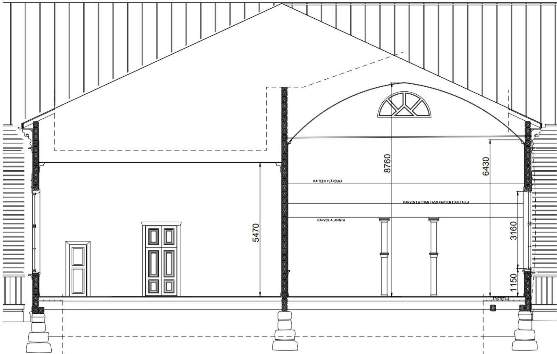
Leikkaus sakariston (vas.) ja pohjoisen sakaran (oik.) kohdalta 2023 tilanteessa mitoilla kohdista, joihin viitataan inventaariossa vuodelta 1836. Mittauspiirustus Elo Sødergren arkkitehdit Oy.
